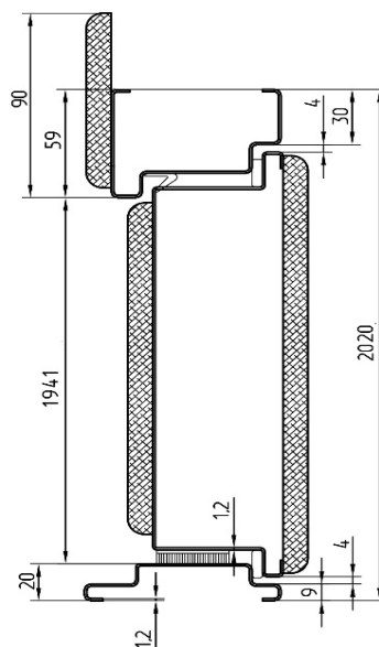
Tehnične dimenzije
